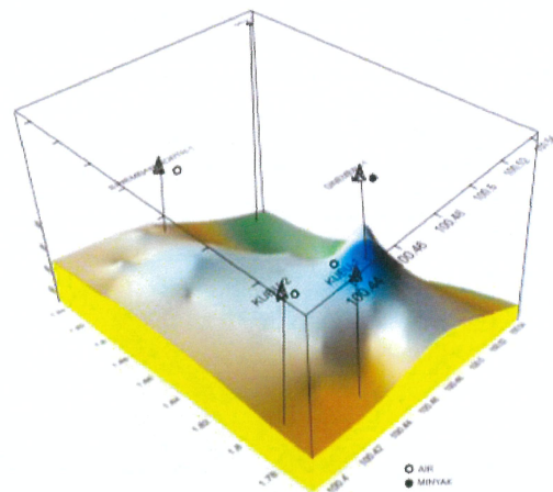
Peta Struktur Geologi bawah permukaan model Pseudo 3D berdasarkan pemetaan time struktur seismik formasi Petani
