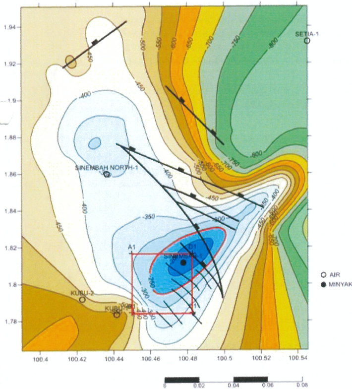
Peta Struktur Geologi bawah permukaan model 2D berdasarkan pemetaan time struktur seismik formasi Petani
